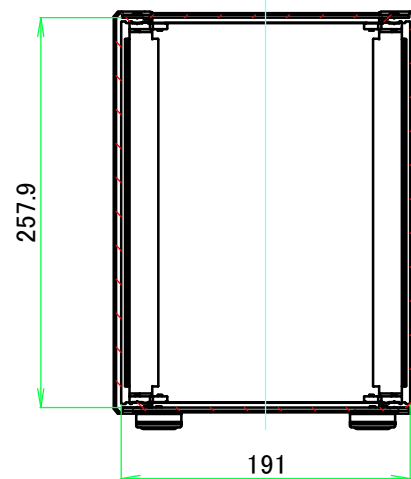
A-A (1:5)
